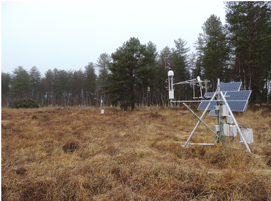
Station Eddy-covariance LICOR LI-7200RS de la tourbière de la Guette.
